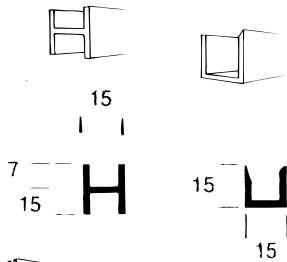
Seitenprofil
